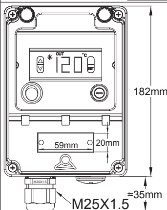
Elektronik-Temperaturregelung mit Digitalanzeige
