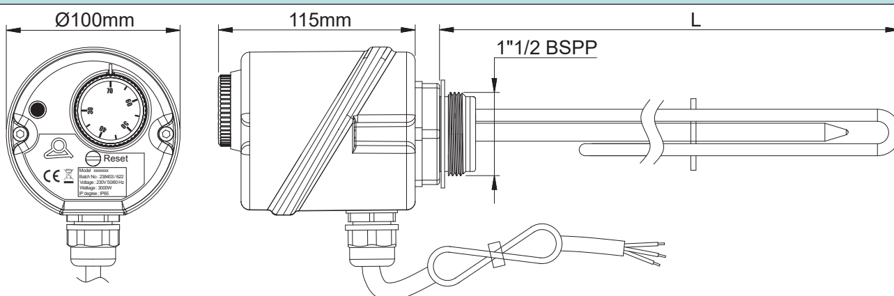
1-poliger 230V-Heizer
