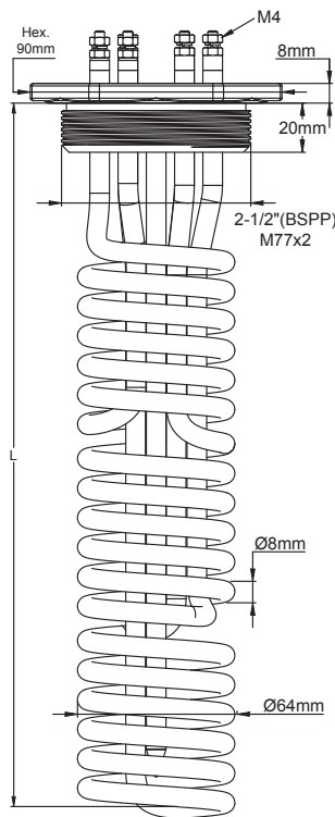
Mit Anschlüssen 2½" BSPP und M77x2
