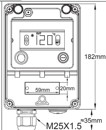
Elektronik-Temperaturregelung mit Digitalanzeige und manuell rückstellbarem Sicherheitsthermostat
